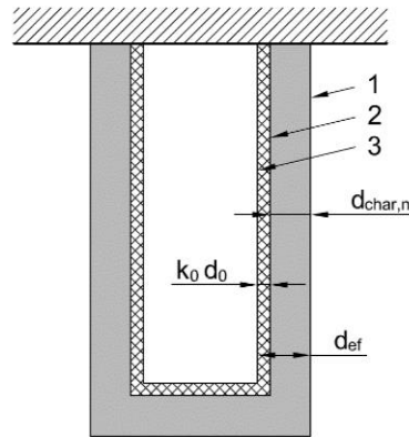
Figura: Definizione di sezione trasversale residua e sezione trasversale efficace. 1 – Superficie iniziale dell'elemento, 2 - Limite della sezione trasversale residua, 3 – Limite della sezione trasversale efficace.
